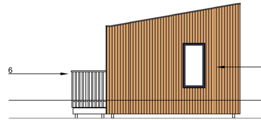
RHS ELEVATION
